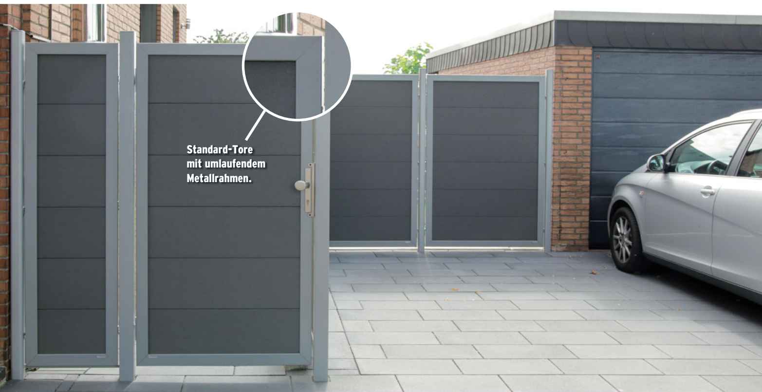
Art. 2280 DESIGN WPC ALU Tor in Anthrazit, DIN rechts, Metallrahmen in Silber, Toraufhängung innen.
